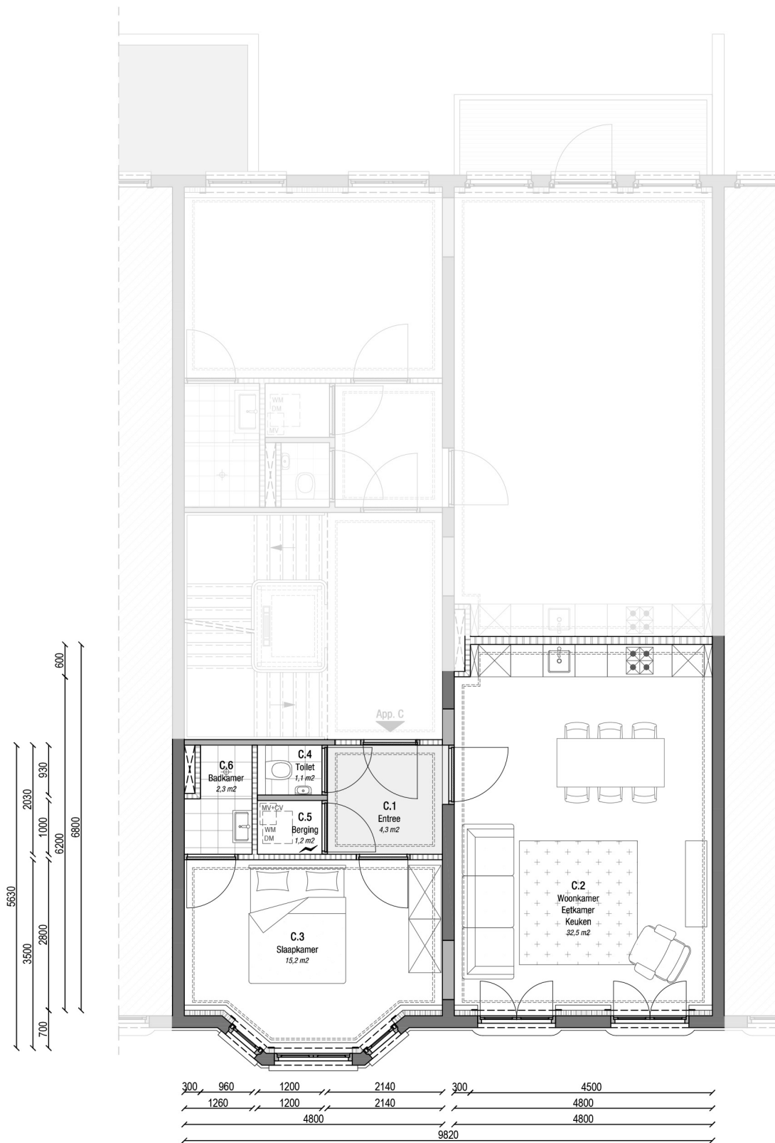
Appartement C eerste verdieping de getoonde maatvoering is indicatief
