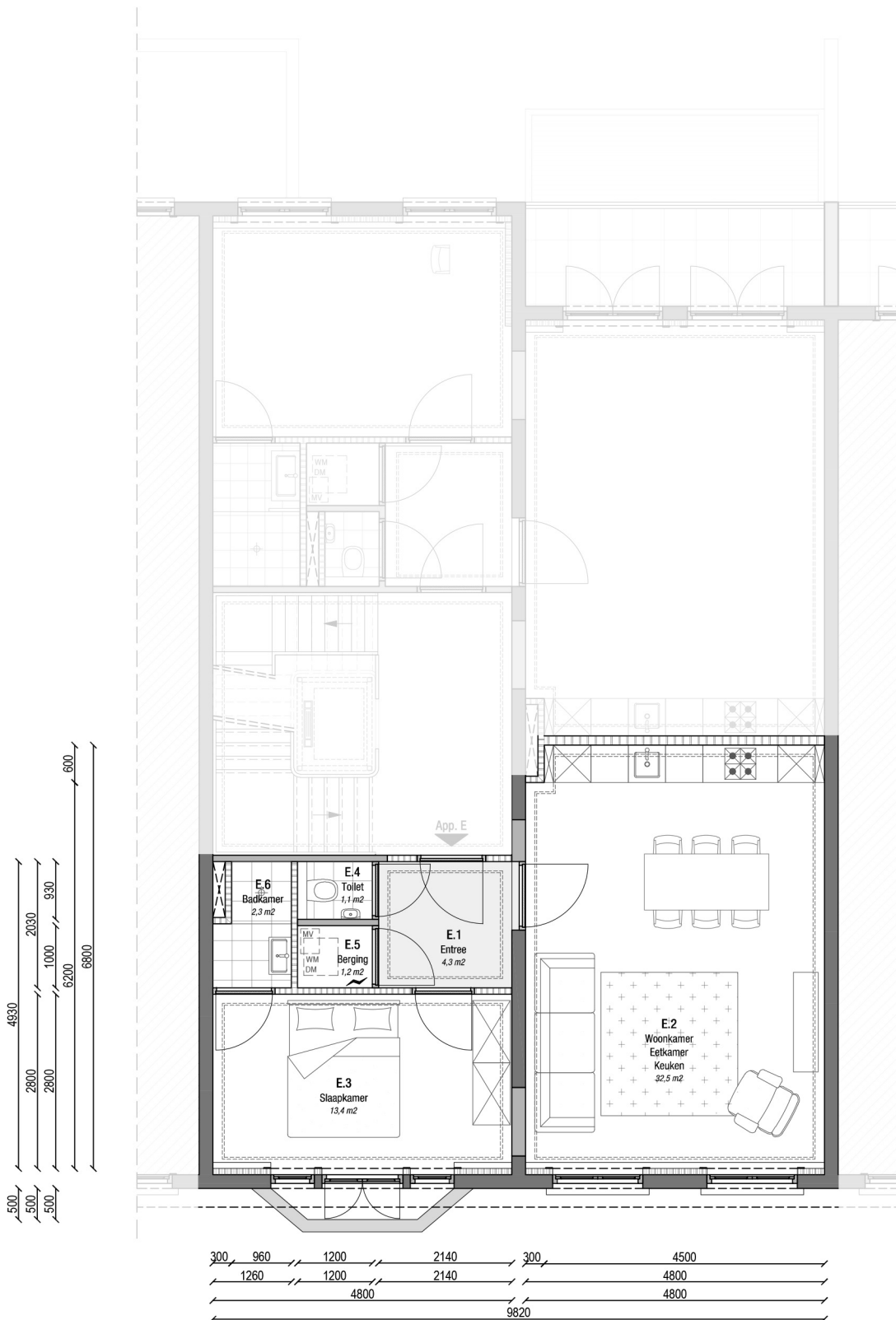
Appartement E tweede verdieping de getoonde maatvoering is indicatief
